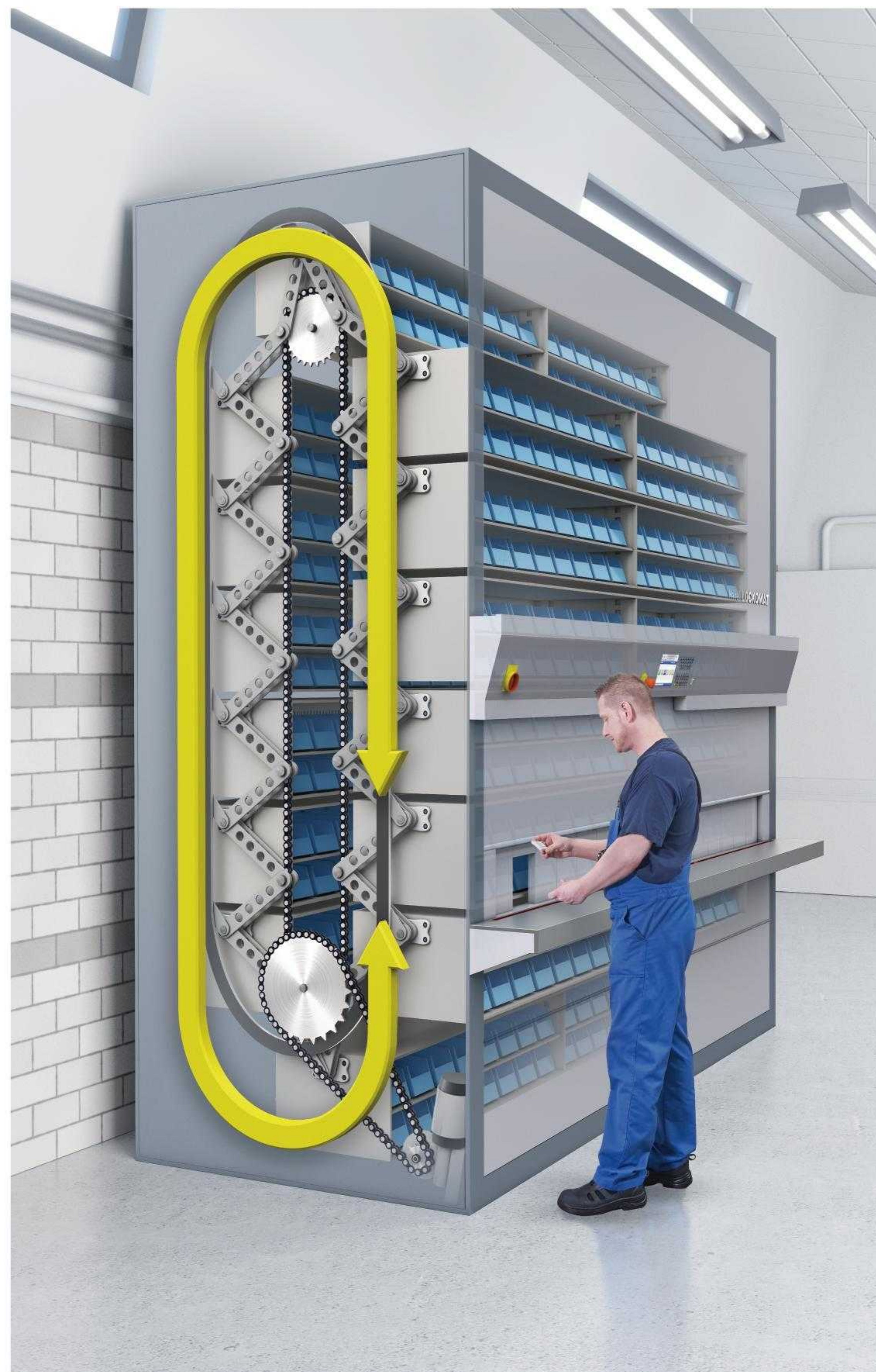
■ HANEL保密旋转柜原理图
